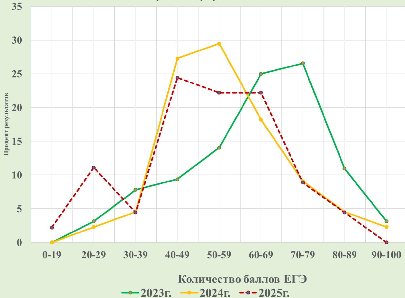
Распределение результатов ЕГЭ
